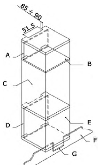
Рис.9: Требования к вентиляции и зазору для установки электрической печи в кухонном шкафу.
